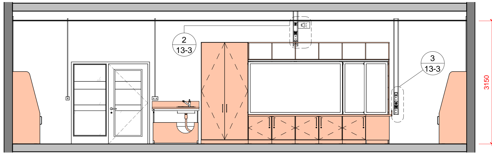
1 Elevation AA 1 : 50
