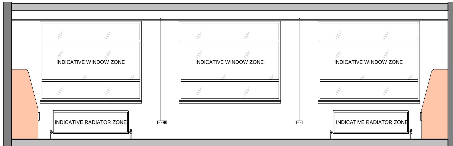
2 Elevation BB 1 : 50
