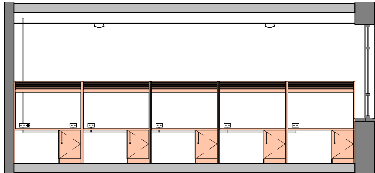
2 Elevation BB 1 : 50
