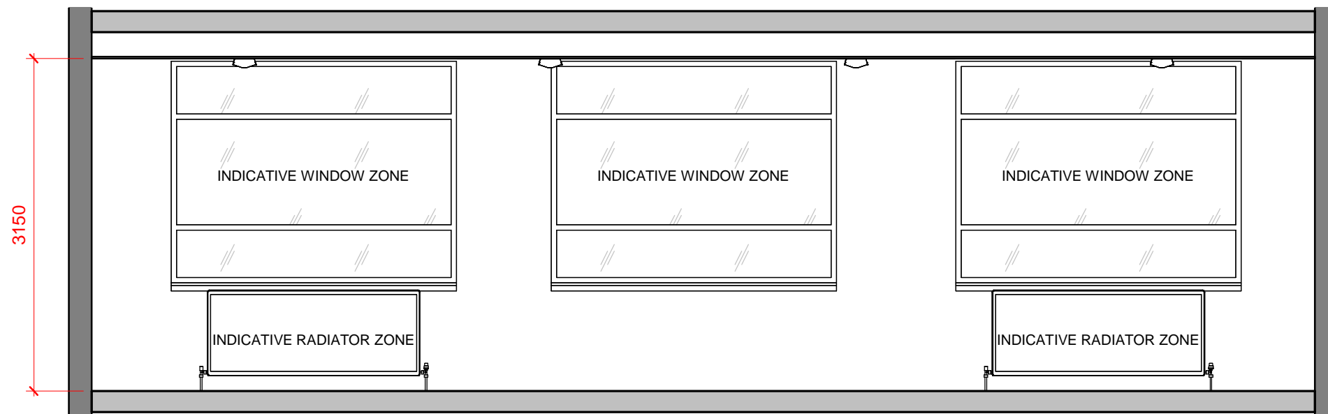
3 Elevation DD 1 : 50
