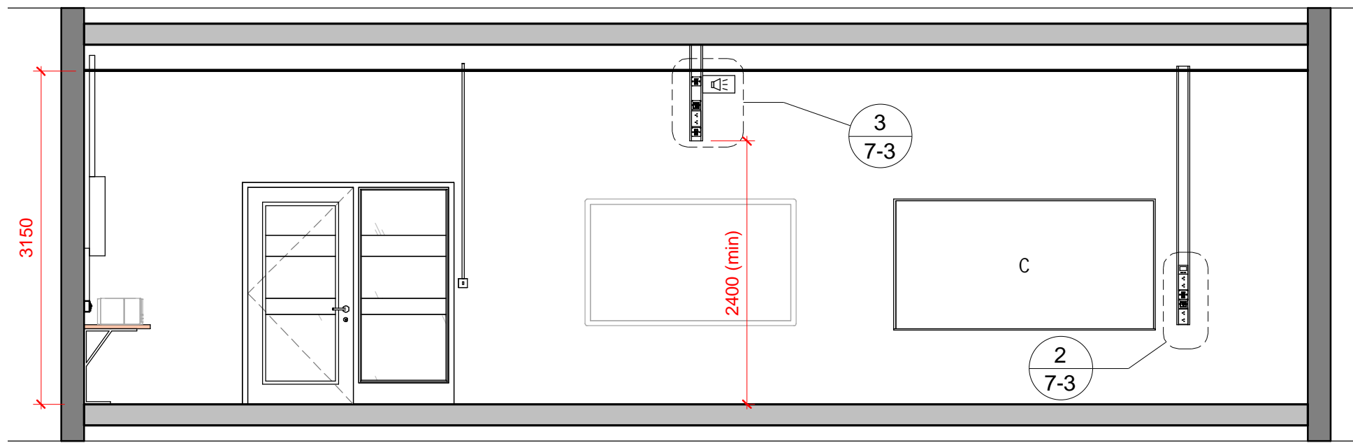
1 Elevation AA 1 : 50
