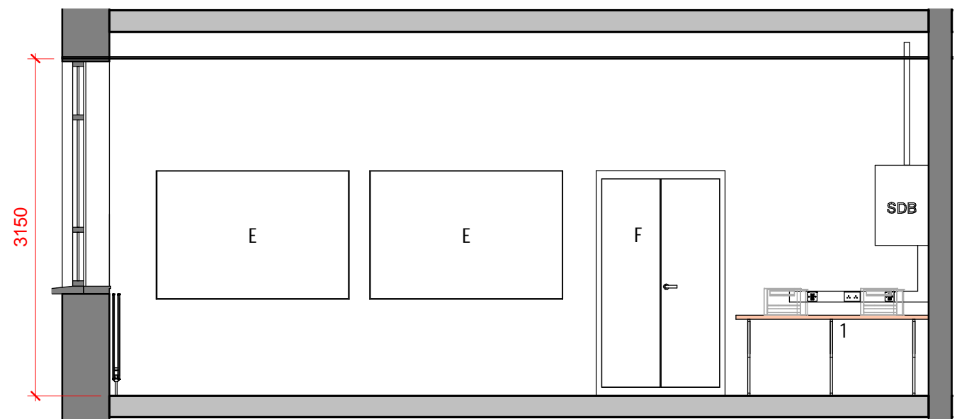
3 Elevation DD 1 : 50
